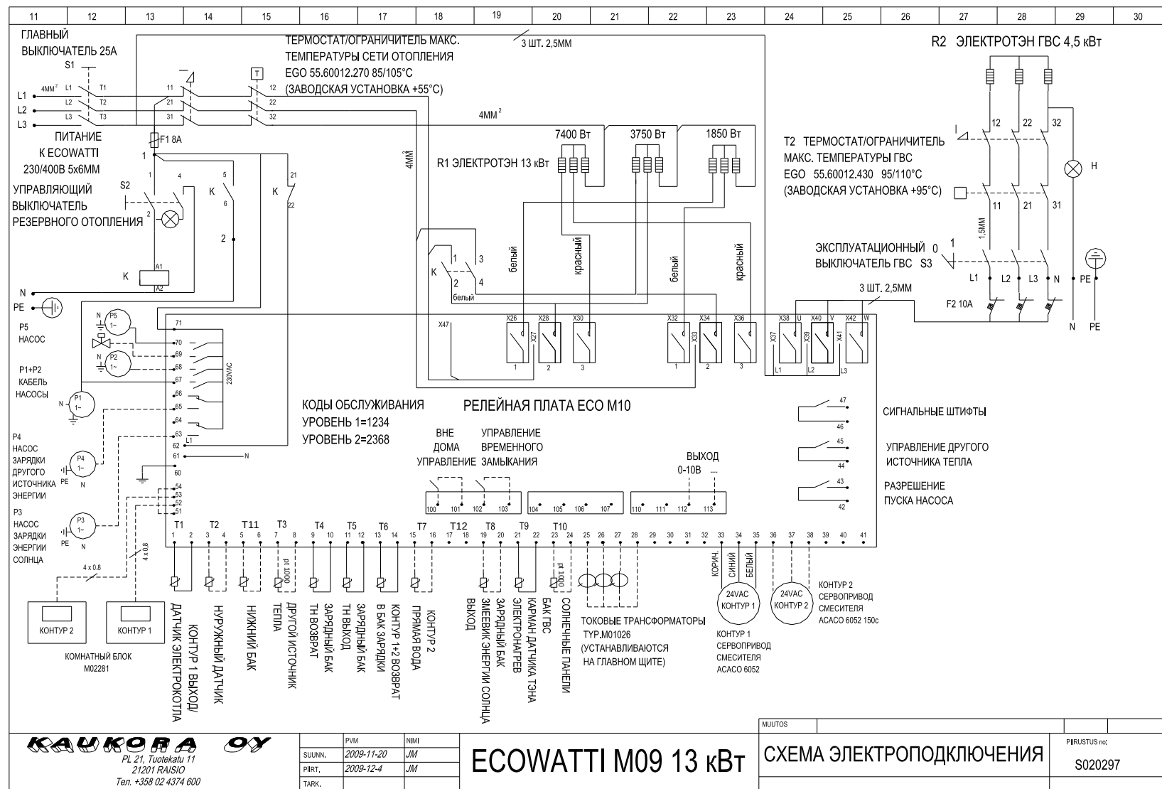
Рис. 8 Схема электроподключения
