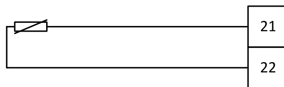
Рисунок 5.11. Схема подключения зонда наружной температуры к электрическому щиту.
